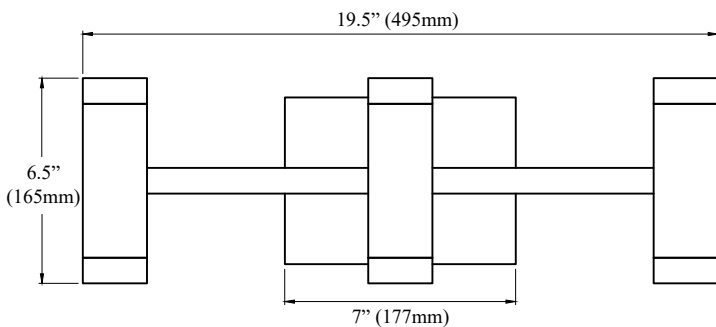
Front Vie/Vue de Face
