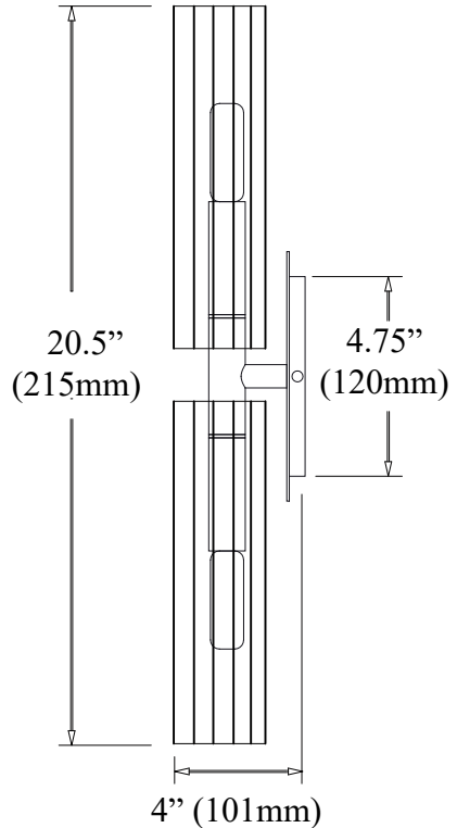
Side View/Vue de Côté
