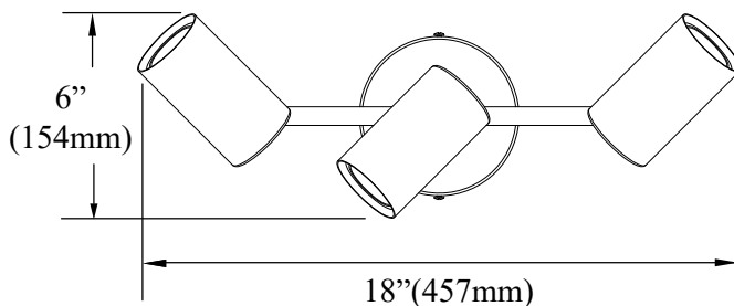
Bottom View/vue de dessous
