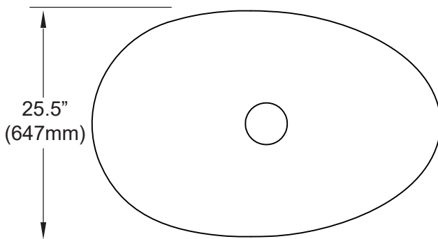
Bottom View / Vue de dessous
