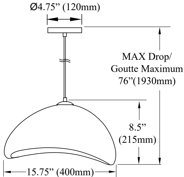
Side View / Vue latérale
