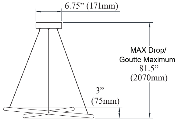
Front view Vue de face
