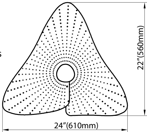
Bottom View/ Vue de dessous
