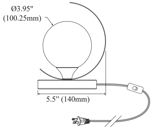
Side view Vue de côté
