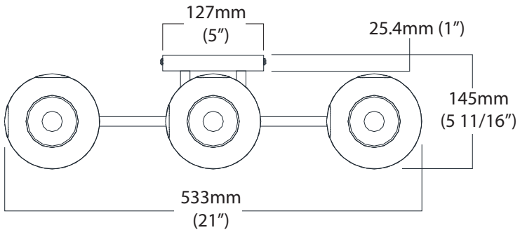
Top View / Vue de Dessus
