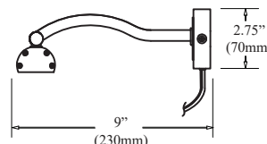
Side View/Vue de Côté
